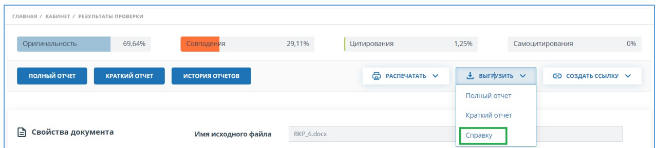
Рисунок 92. Кнопка «Справка»
