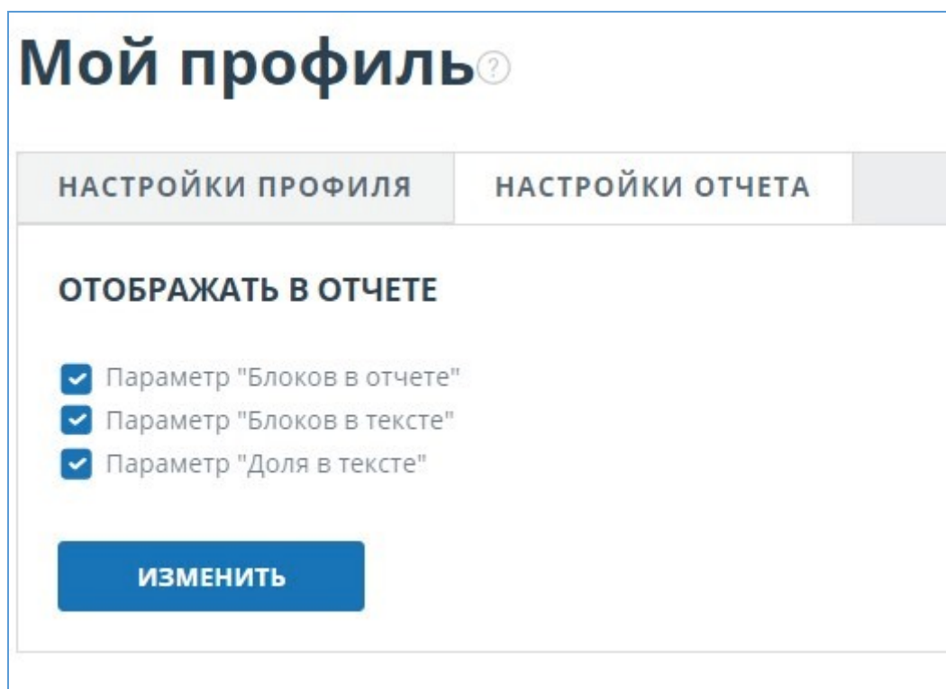
Рисунок 11. Настройки отчета
