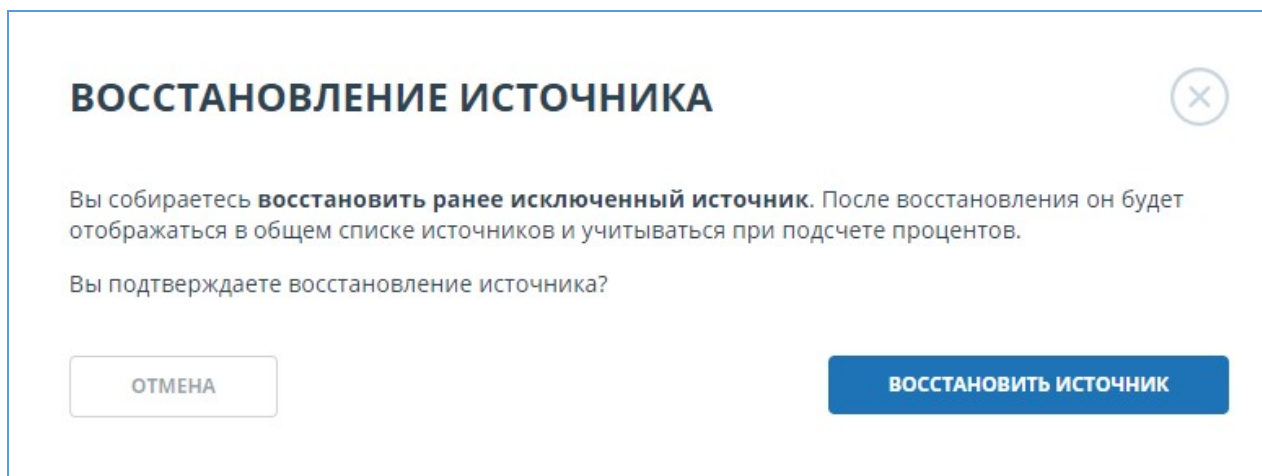
Рисунок 57. Подтверждение восстановления
