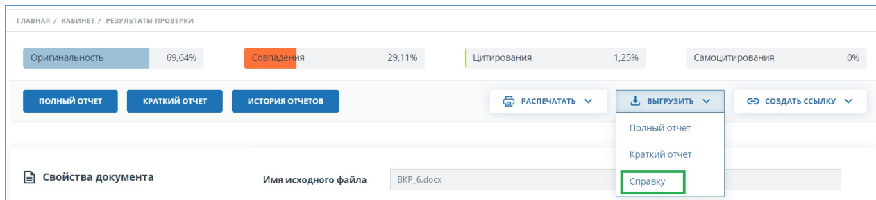
Рисунок 92. Кнопка «Справка»
