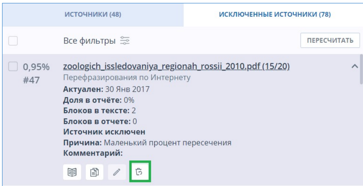
Рисунок 56. Восстановление источника
