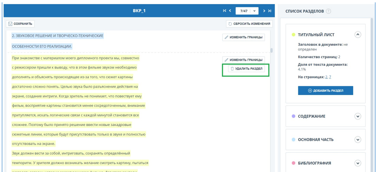
Рисунок 76. Удаление раздела
