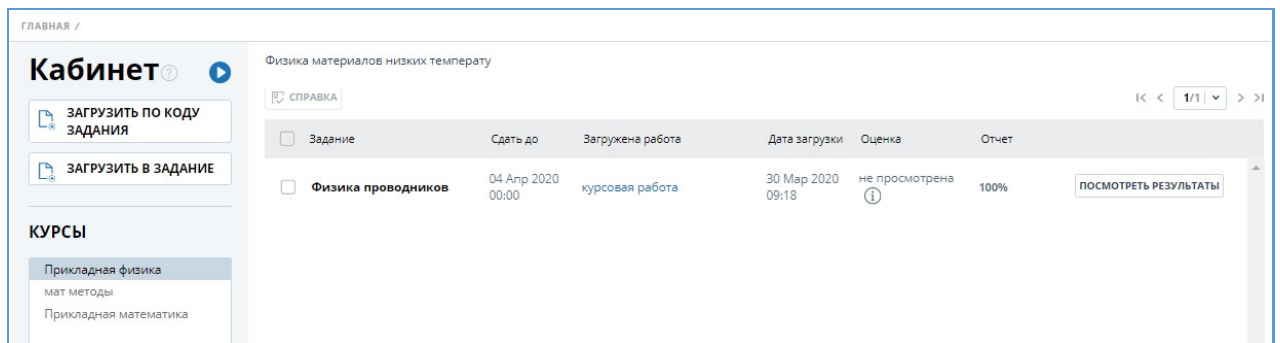
Рисунок 8. Кабинет студента
